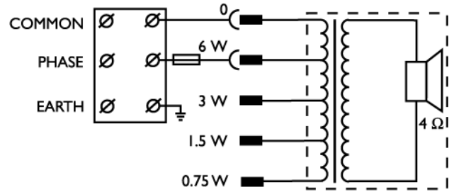
Принципиальная схема
