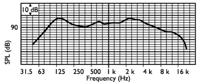
Частотная характеристика
